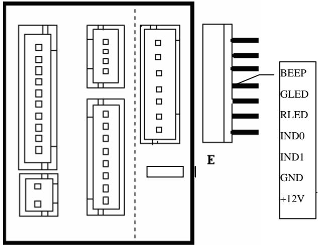
有 Weigend 输入接线排插座定义
